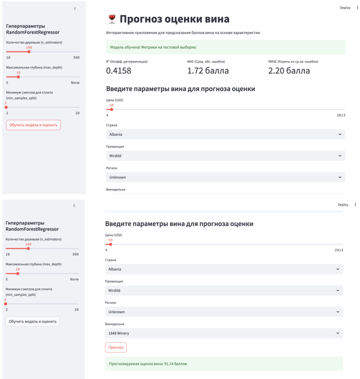
Рисунок 14 – Веб-приложение.
